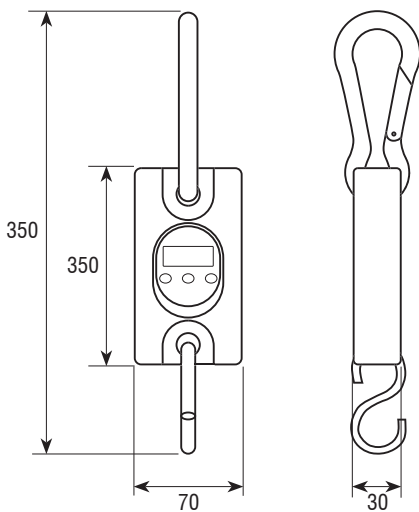
Dimensions en mm
